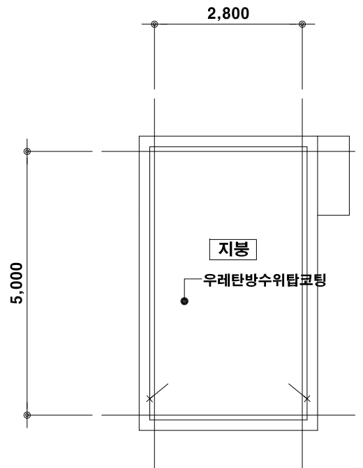
욕탑지붕 평 면 도 scale:1/100
